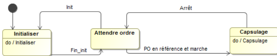
Diagramme d'états de la capsuleuse de bocciaux
