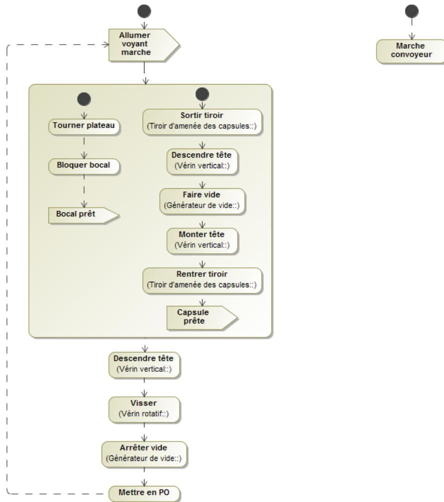
Diagramme d'activité du capsulage de la capsuleuse
