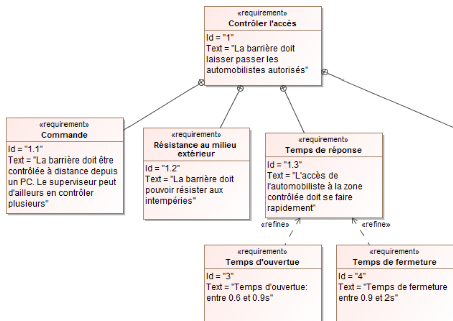
Diagramme des exigences (partiel) de la barrière Sympact
